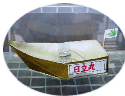
ポンポン船
