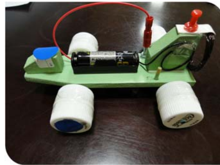
電磁力推進車
