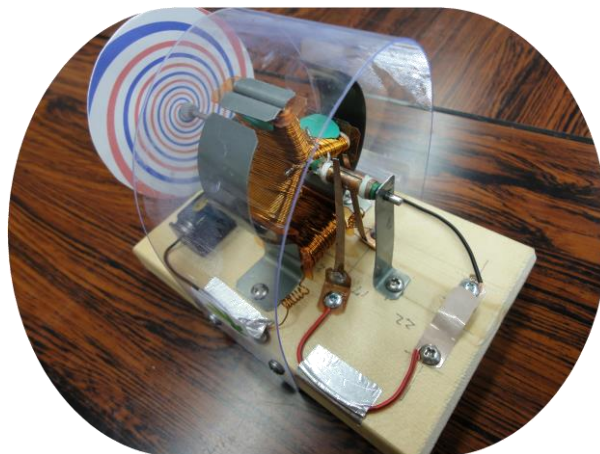
3極直流モーター
