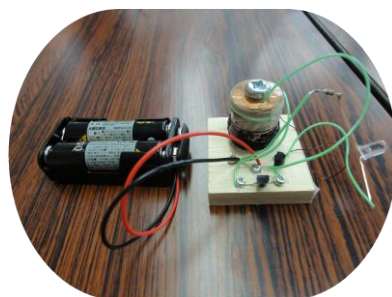
ボックスに収納の 電磁石
