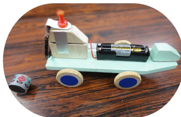
電源入切にリードスイッチを使用した 電磁力推進車
