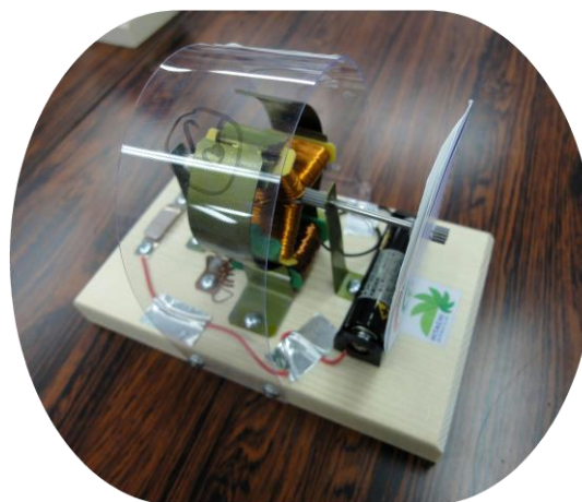
3極直流モーター
