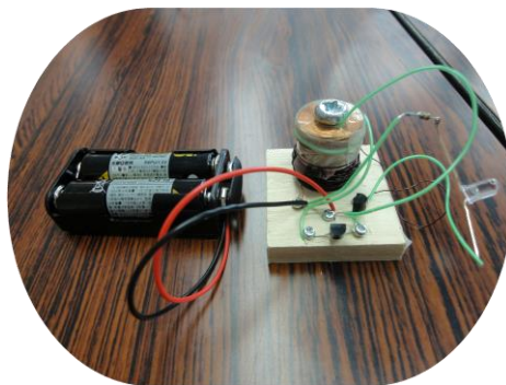
ボックスに収納の電磁石
