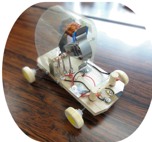
電磁石エンジン
