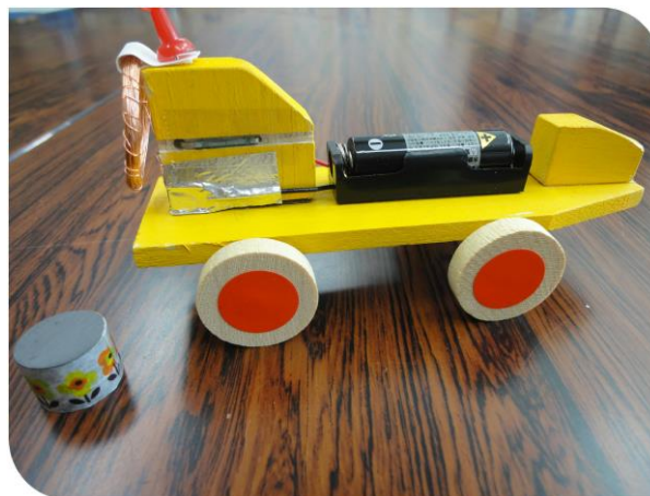
電磁力推進車
