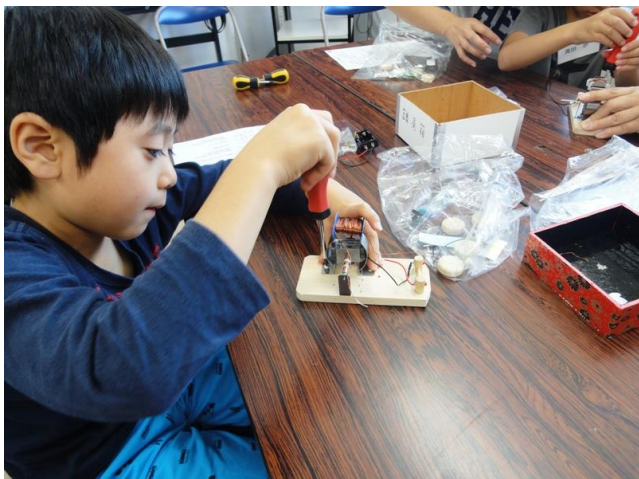
固定子側電磁石組みこみ
