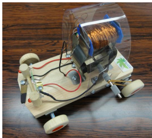
ハイパワー電磁石エンジン
