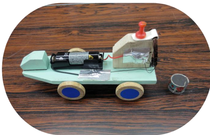
電磁力推進車
